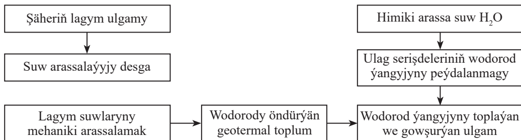
Shema. Ýaşyl wodorody lagym suwlaryndan öndürmegiň tehnologiýasy
