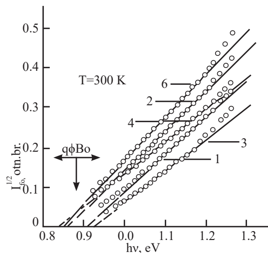
2-nji surat. I_0^{1/2} - h\nu koordinatada 5 sany Pd-n-GaAs strukturalaryň fototogunyň spektri we ol deň sanly fotonlaryň düşüşine normirlenen.
