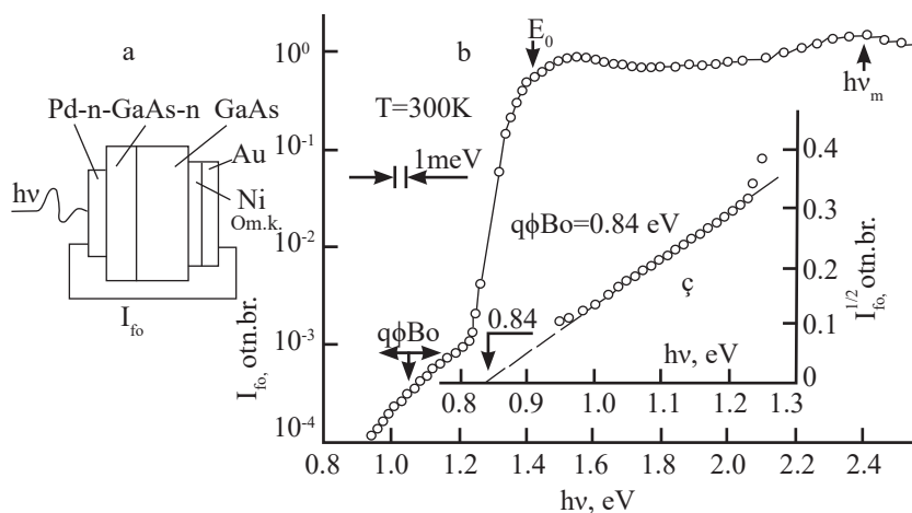
1-nji surat. Diodyň gurluşynyň we gysga utgaşdyрма fototogunyň I_0 ölçenilişiniň shemasy (a) we Pd-n-GaAs strukturanyň fototogunyň ( I_0 ) fotonyň energiýasyna ( h\nu ) baglylygy (b).
