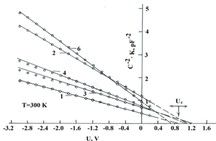
3-nji surat. C^{-2}-U koordinatada 5 sany Pd-n-GaAs strukturalaryň sygymynyň (c) naprýaženiýa (U) baglylygy.
